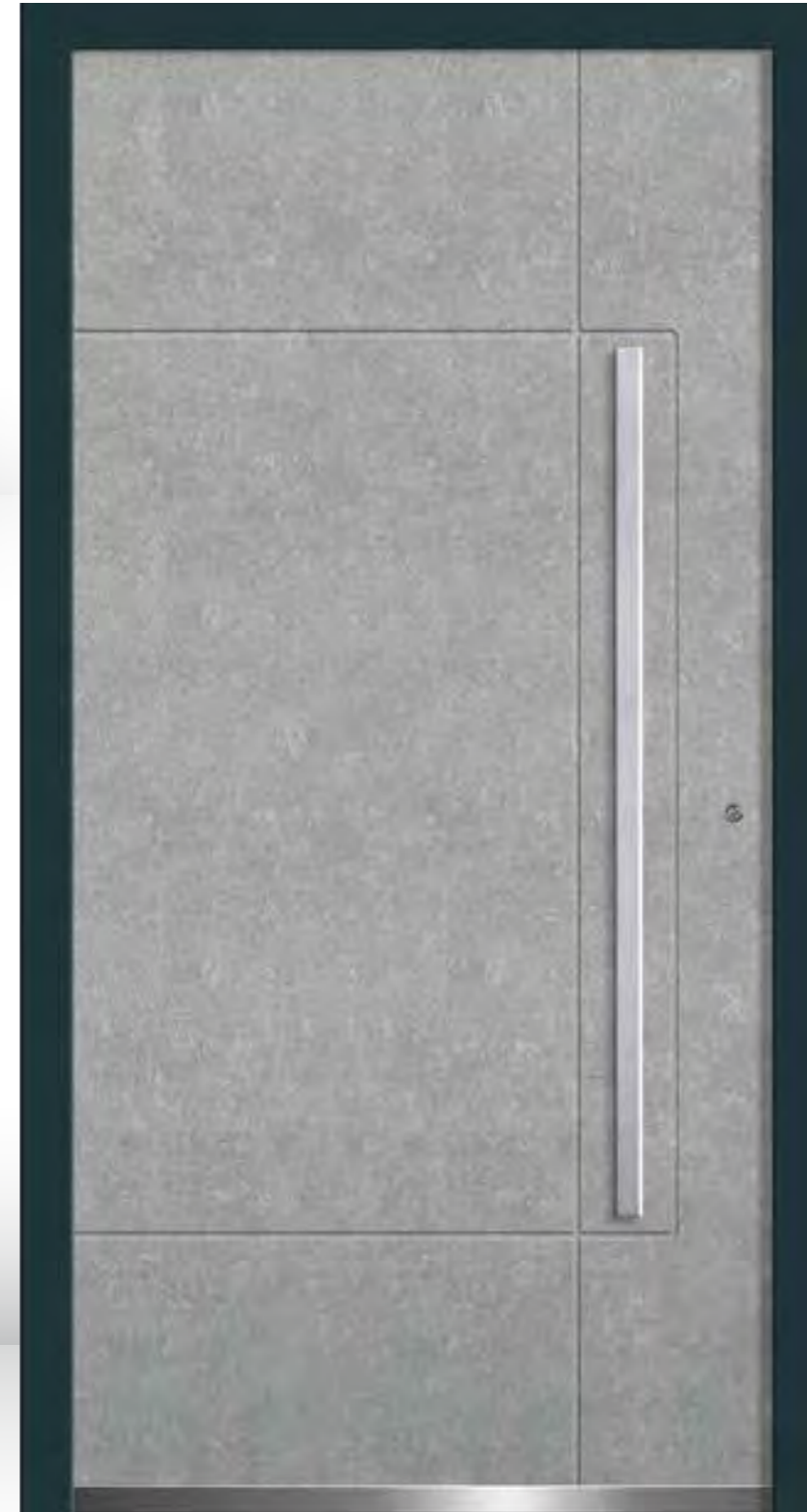
M-490 D Ansicht A / DIN rechts Flachnuten außen ■ Aufsatzfüllung ■ Designoberfläche Concrete ■ Griff ZAE 147 | PG 11 ■ flächenbündiger Trittschutz TS 7
